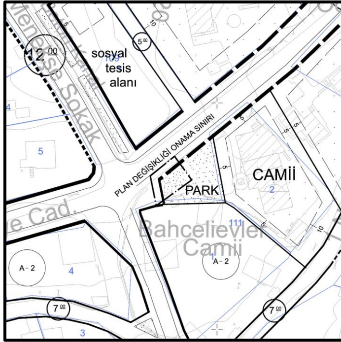
Şekil 2. Trafo Alanına Ait 1/1000 Ölçekli Mevcut Uygulama İmar Planı
