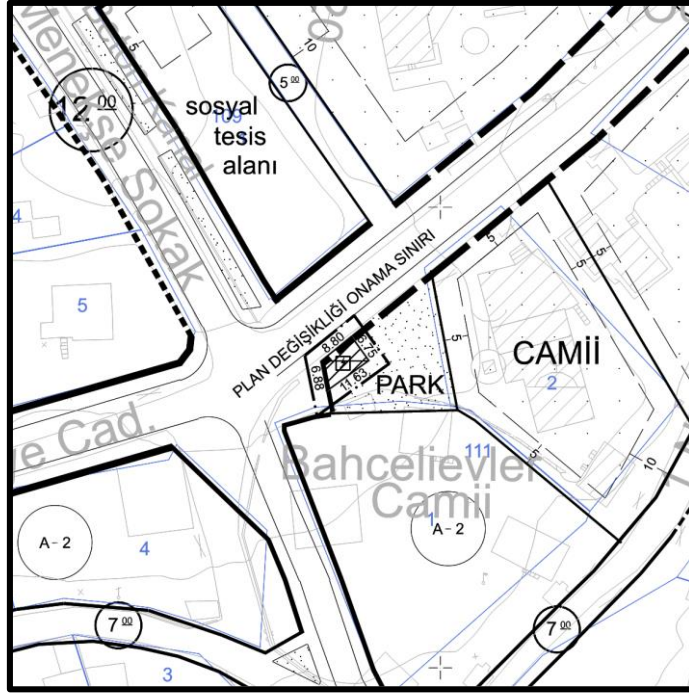
Şekil 3. Trafo Alanına Ait 1/1000 Ölçekli Uygulama İmar Planı Değişikliği
